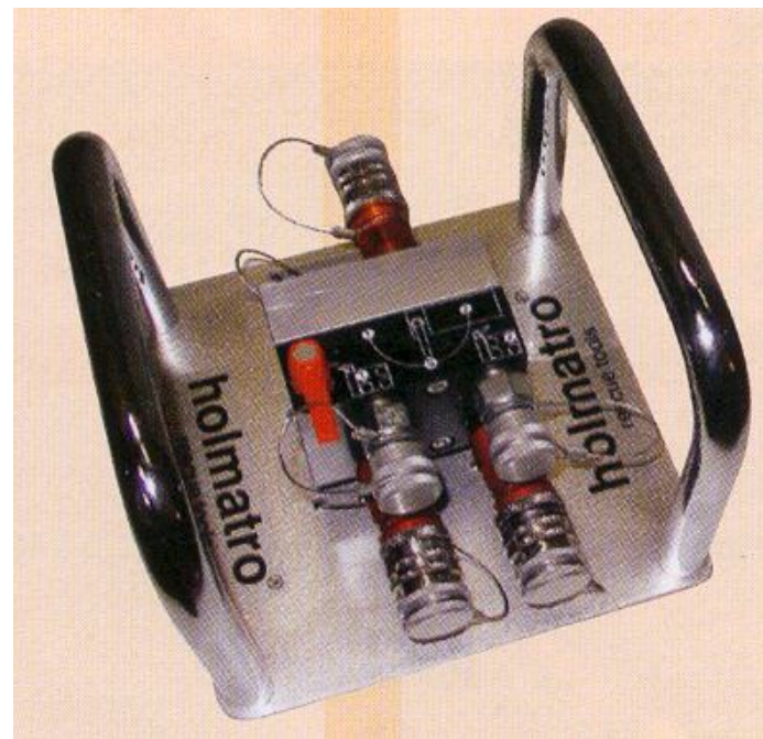
Rozdzielacz systemu jednowężowego
